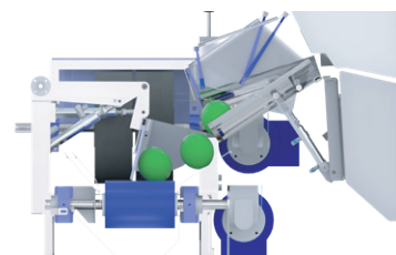
Taśmociąg poprzeczny
